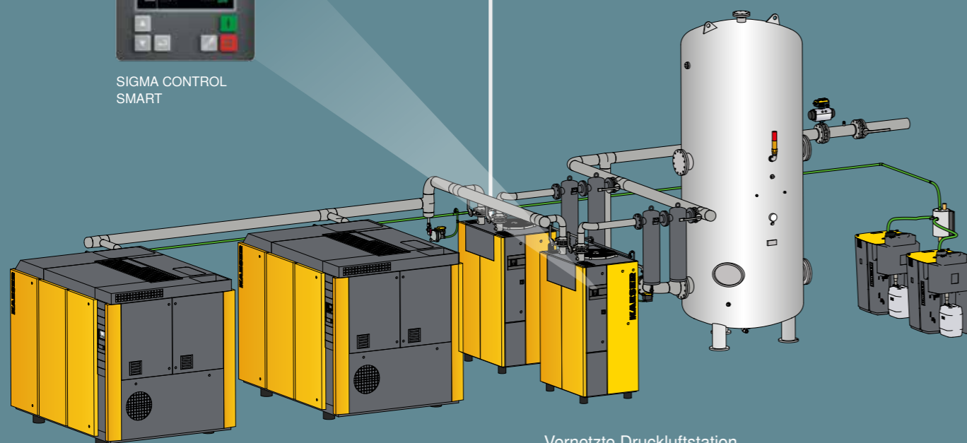
Vernetzte Druckluftstation
