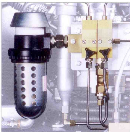
Kondensatautomatik
